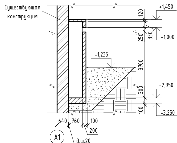
2-2 Опалубка
