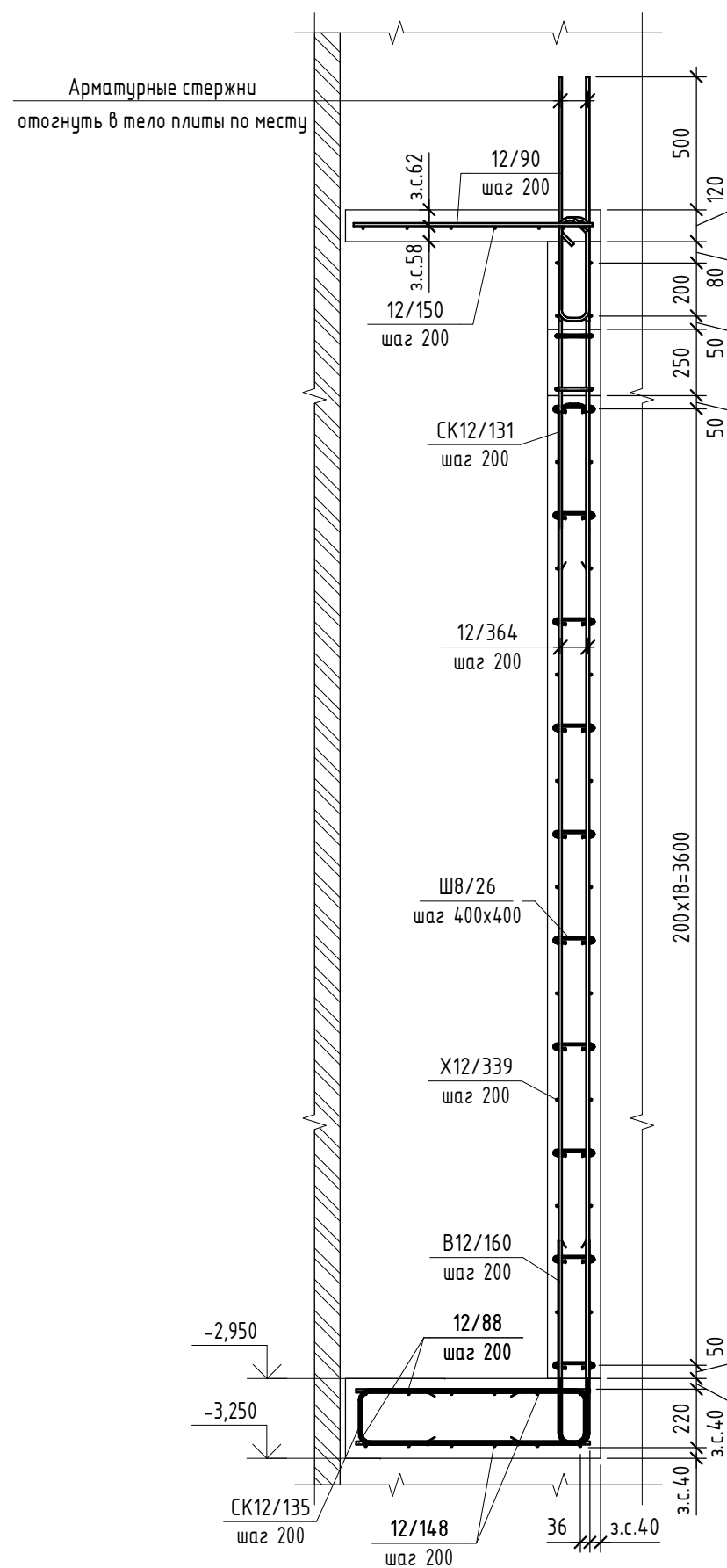
2-2 Армирование
